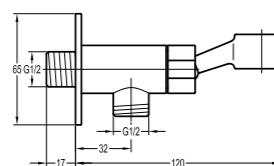
FH 8853E 全铜万向支架 · 光亮铬
