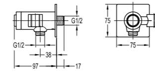
FH 8817A 全铜淋浴器接头 (按键式) · 带花洒支架 · 光亮铬
