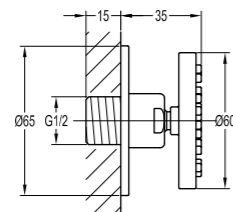
FH S27B 淋浴侧喷 · 1/2"管接 · 光亮铬
